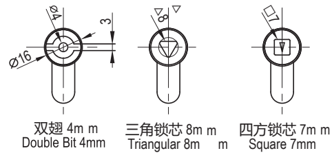
挂锁装置 Padlock device
