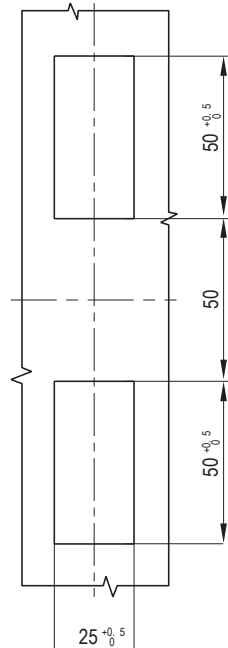
开孔尺寸 Panel Cutout
