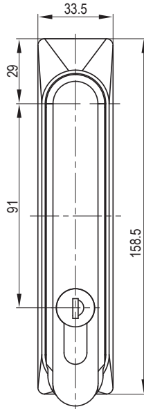
半圆柱 K333 相同钥匙 Alike K333 Proble Round Cylinder
