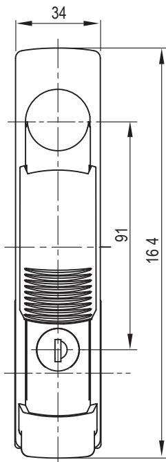
圆柱 K333 相同钥匙 Alike K333 Round Cylinder
