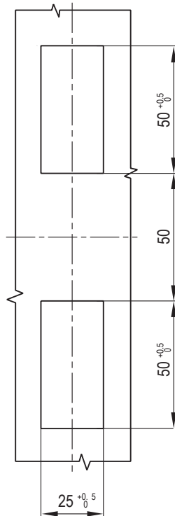
开孔尺寸 Panel Cutout
