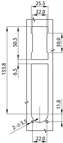
开孔尺寸 Panel cutout
