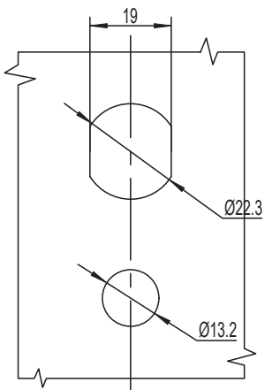
开孔尺寸
