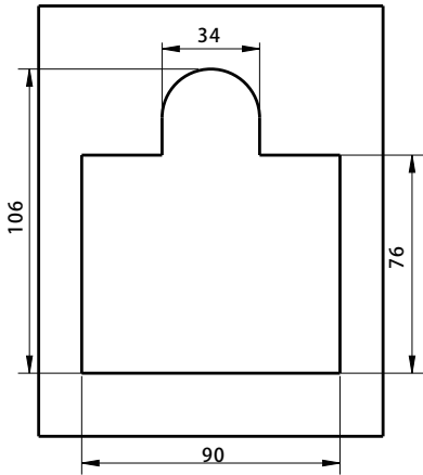
开孔尺寸 Panel Cutout
